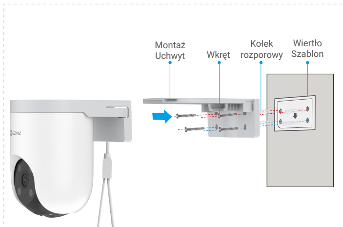
Rys. 2 Montaż ścienny
