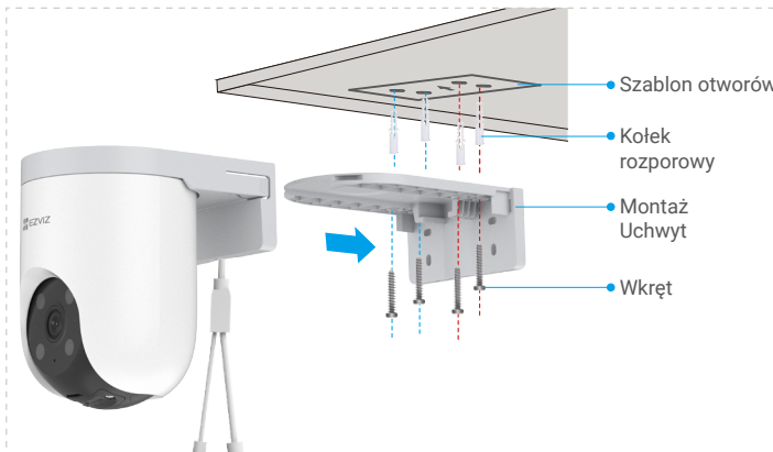
Rys. 1 Montaż sufitowy
